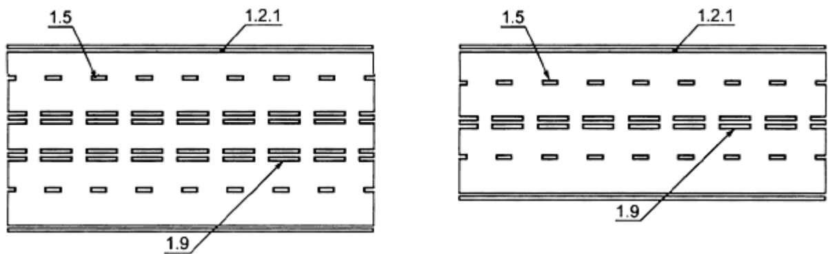
Рисунок В.16 - Примеры нанесения разметки 1.9
