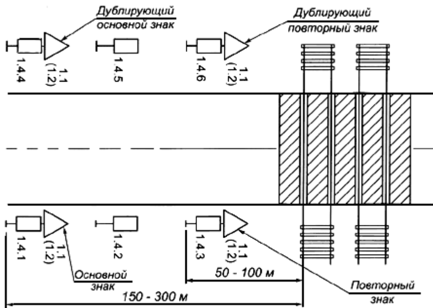
Рисунок В.3 - Размещение знаков 1.4.1-1.4.6
