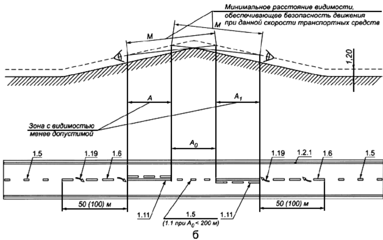
Рисунок В.6 - Примеры нанесения разметки на участках дорог с
